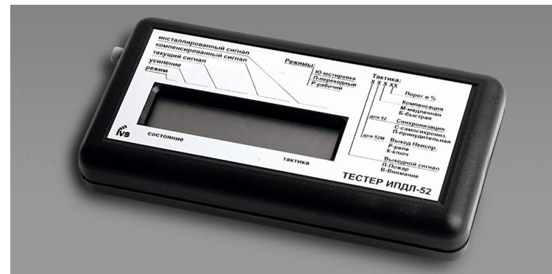
Тестер ИПДЛ-52 Пусконаладочное и сервисное оборудование
